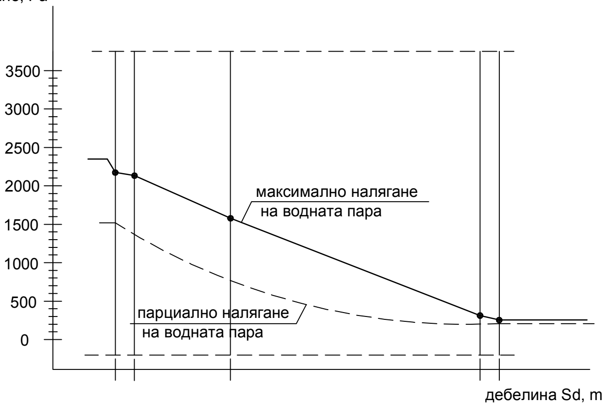
Крива на максималното и парциалното налягане през многослойна ограждаща конструкция
