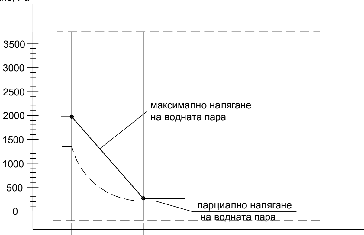
Крива на максималното и парциалното налягане през многослойна ограждаща конструкция
