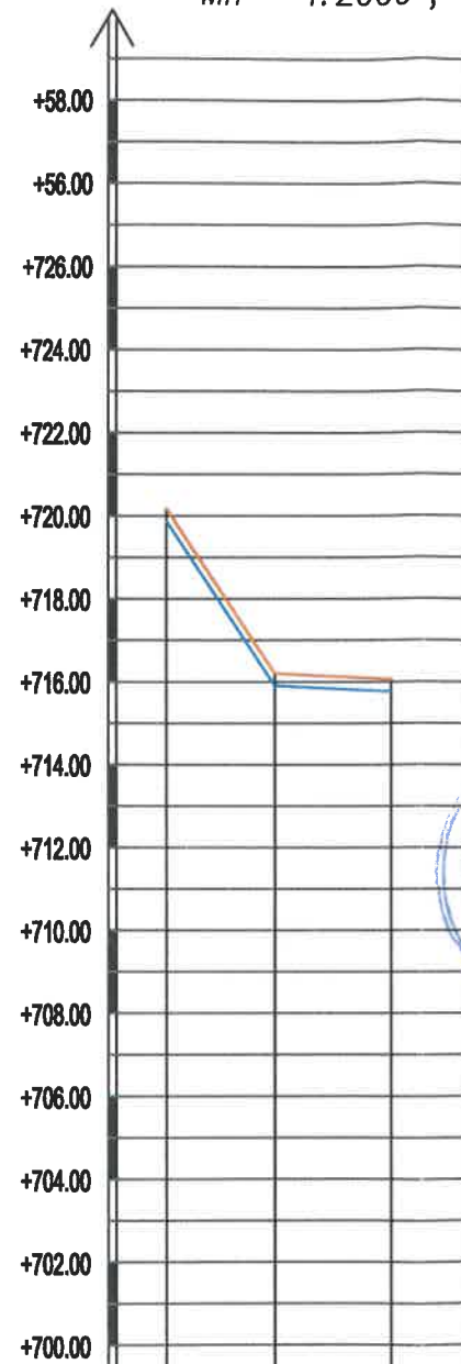
Надлъжен профил на отводнителна канавка кл.2 Mh = 1:2000 ; Mv = 1:200
