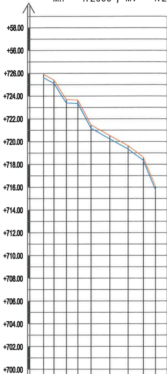
Надлъжен профил на отводнителна канавка кл.1 Mh = 1:2000 ; Mv = 1:200
